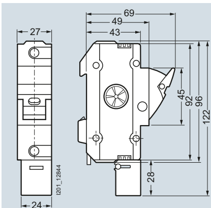
3NC1491-5
