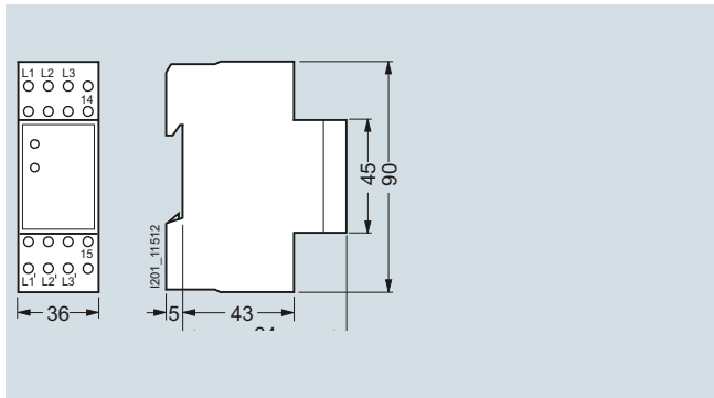
5TT3170
