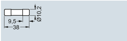
3NC10..
