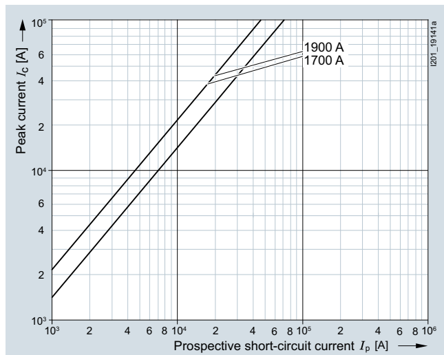
3NB33..-1KK27
