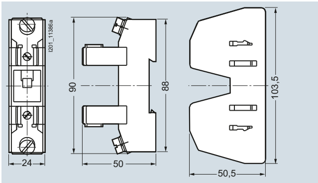
3NC1451-1
