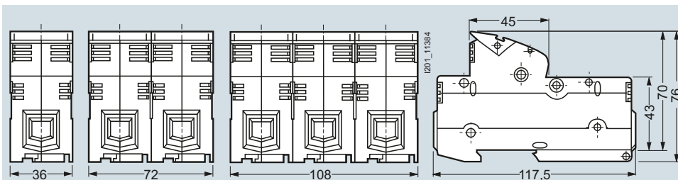
3NC129.
