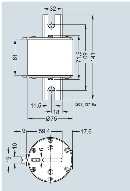
3NC24...-0C, 3NC84...-0C
