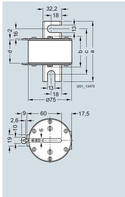
3NC34...-1U
