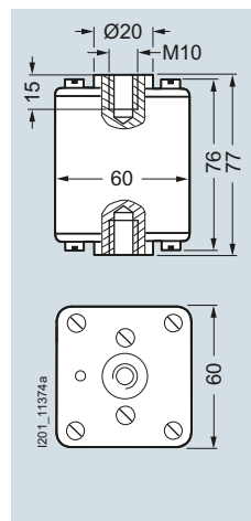
3NE43...-6B, 3NE4337-6
