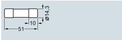
3NC14..
