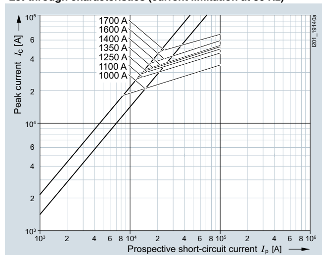
3NB33..-1KK26
