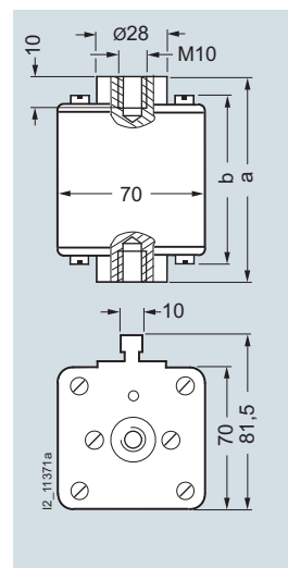
3NE64..., 3NE94...
