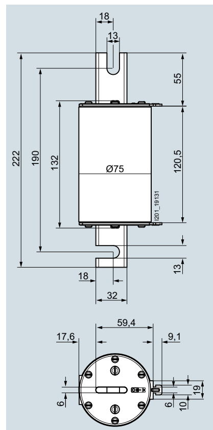
3NB1337-4KK11 3NB1345-4KK11
