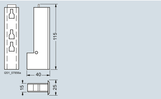
3NX1021
