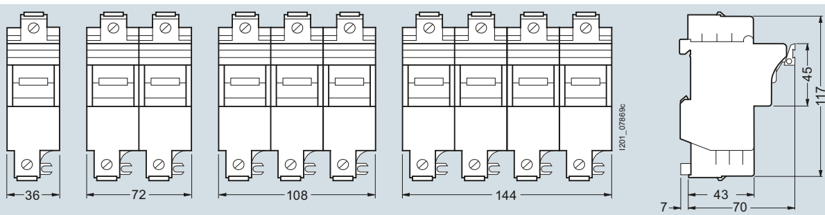
3NW72 1P 1P+N/2P 3P 3P+N
