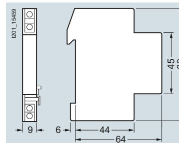
3NW7903
