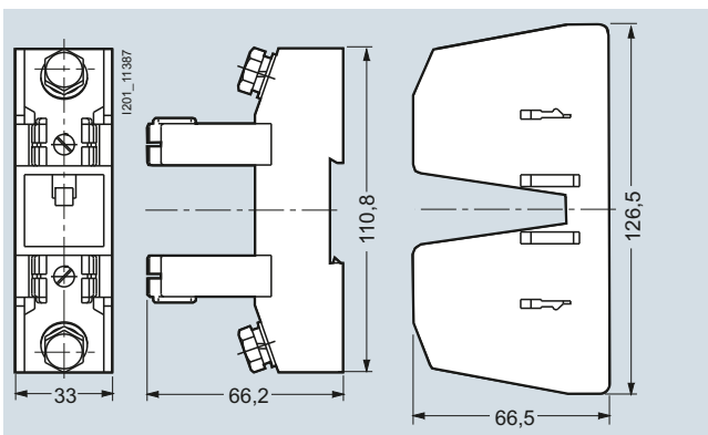
3NC2258-1
