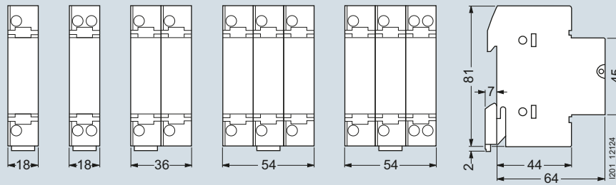
3NW70, 3NW73 1P 1P + N 2P 3P 3P+N
