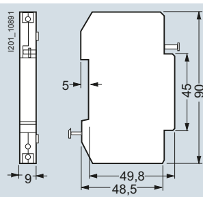
3NW7901 3NW7902
