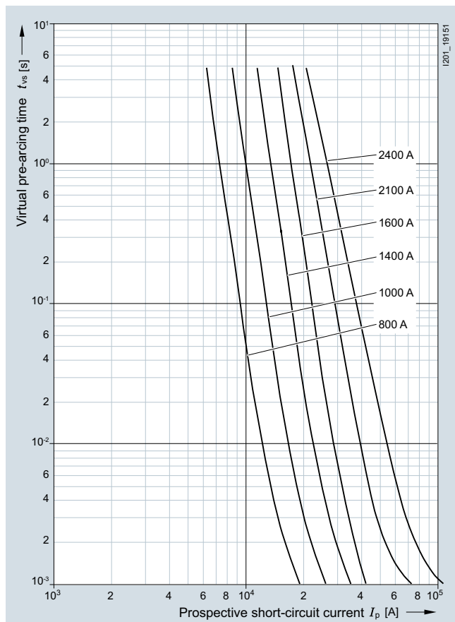
3NB2...-4KK1.
