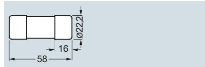
3NC22..
