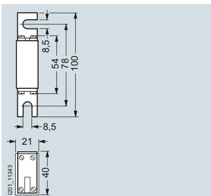
3NE87...-1
