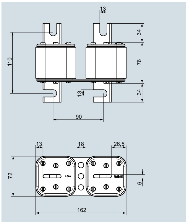
3NB335-1KK26
