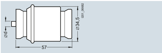
5SD510, 5SD520
