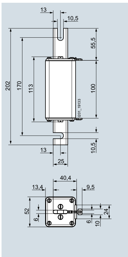
3NB1126-4KK11 3NB1128-4KK11
