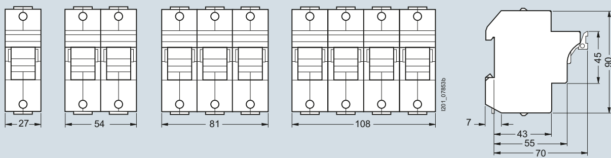
3NW71 1P 1P+N/2P 3P 3P+N
