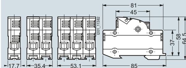
3NC109.
