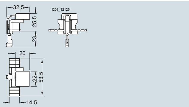
3NX1024
