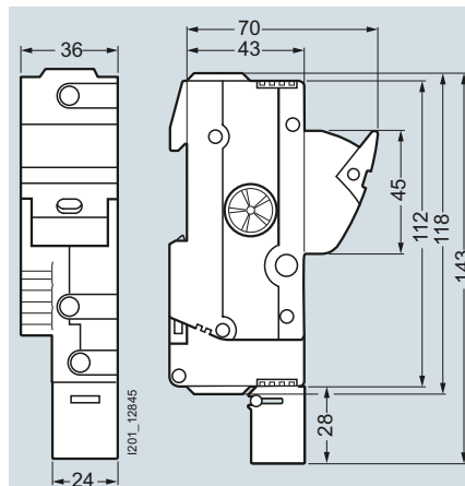
3NC1291-5
