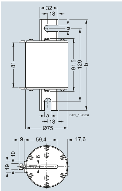
3NE3...-0C, 3NE36...-1C
