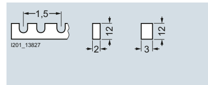
5SH5321 5SH5322
