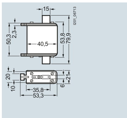
3NE18...-0
