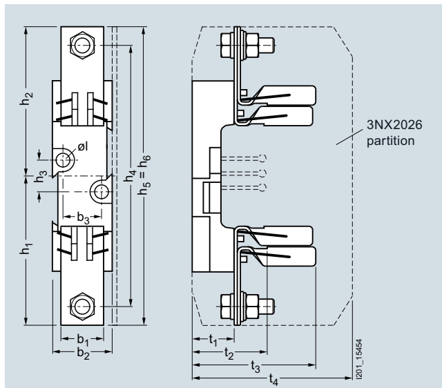
3NH34.0
