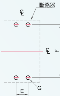
斷路器鑽孔圖
