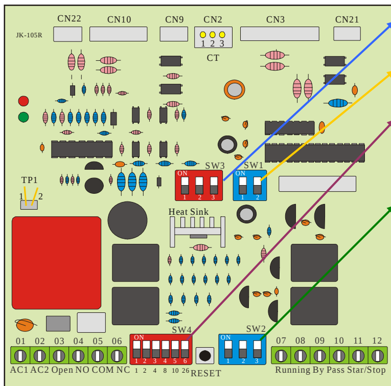
泵浦緩衝器內部示意圖
