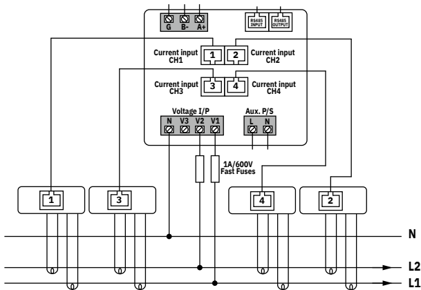
單相三線式電源
