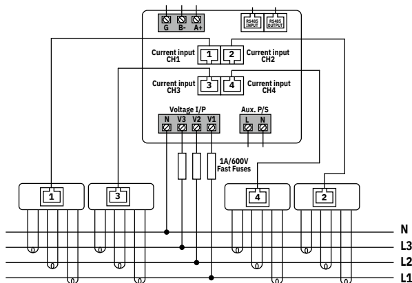
三相四線式電源
