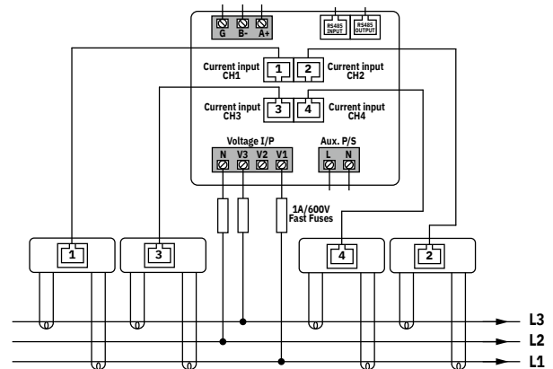
三相三線式電源
