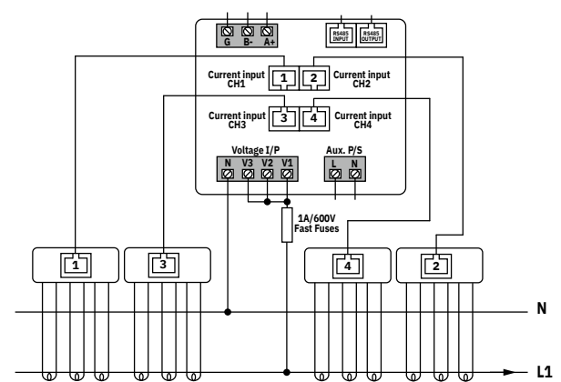
單相二線式電源
