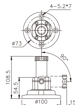
TPTL6-F (新型式專利, 圓形塑膠盤) 使用於TPFS4/TPFF4/TPFB4 TPF□5/TPF□6/TPF□7
